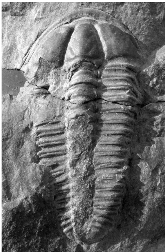
Conocoryphe sulzeri Schlotheim, 1823 †
