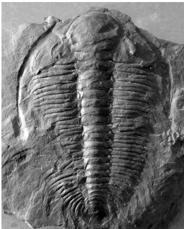
Rejkocephalus rotundatus Barrande, 1846 †
