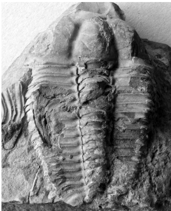
Conocoryphe sulzeri Schlottheim, 1823 †
