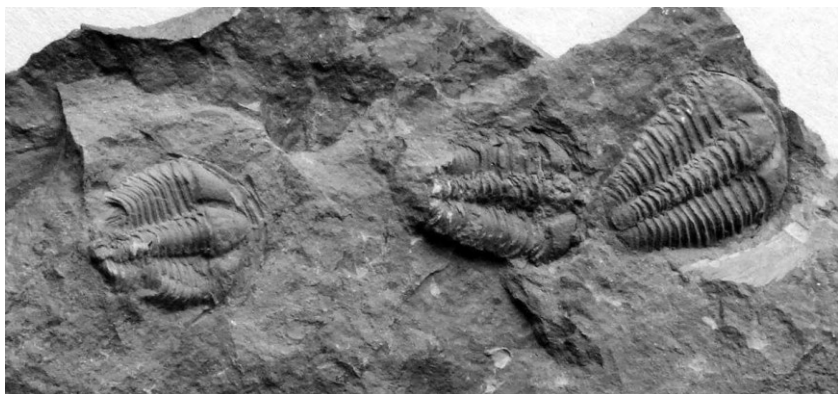
Conocoryphe cirina Šnajdr, 1982 †
