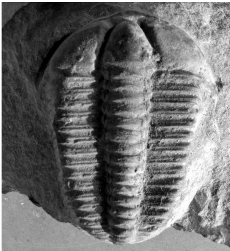
Conocoryphe sulzeri Schlotheim, 1823 †
