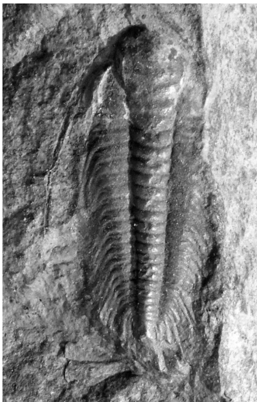
Paradoxides gracilis Boeck, 1827 †
