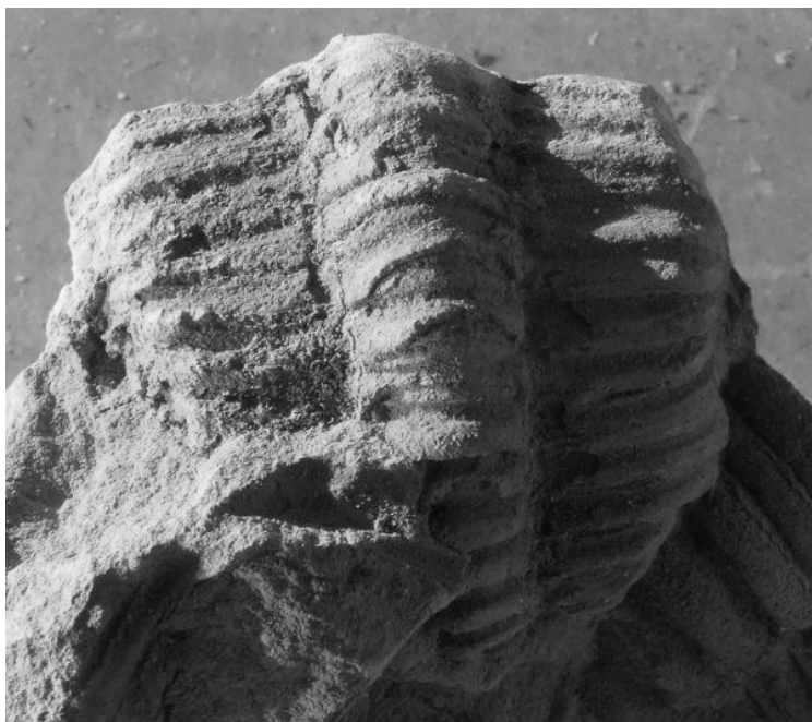
Conocoryphe nanciscor Vokáč, 1997 †
