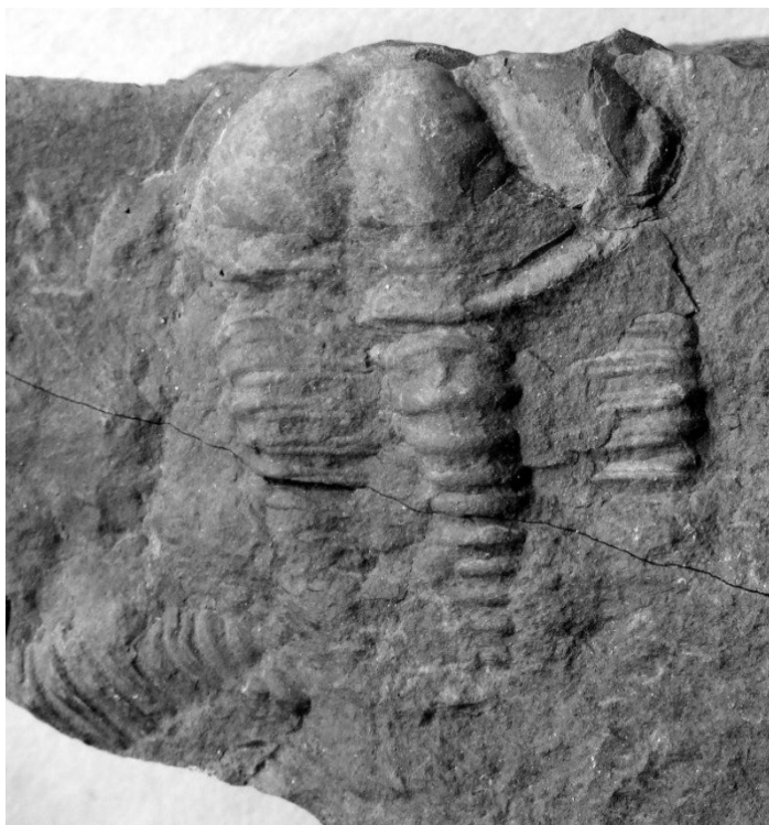
Conocoryphe sulzeri Schlotheim, 1823 †
