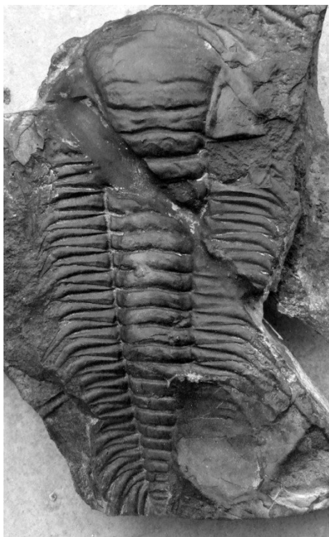
Paradoxides gracilis Boeck, 1827 †
